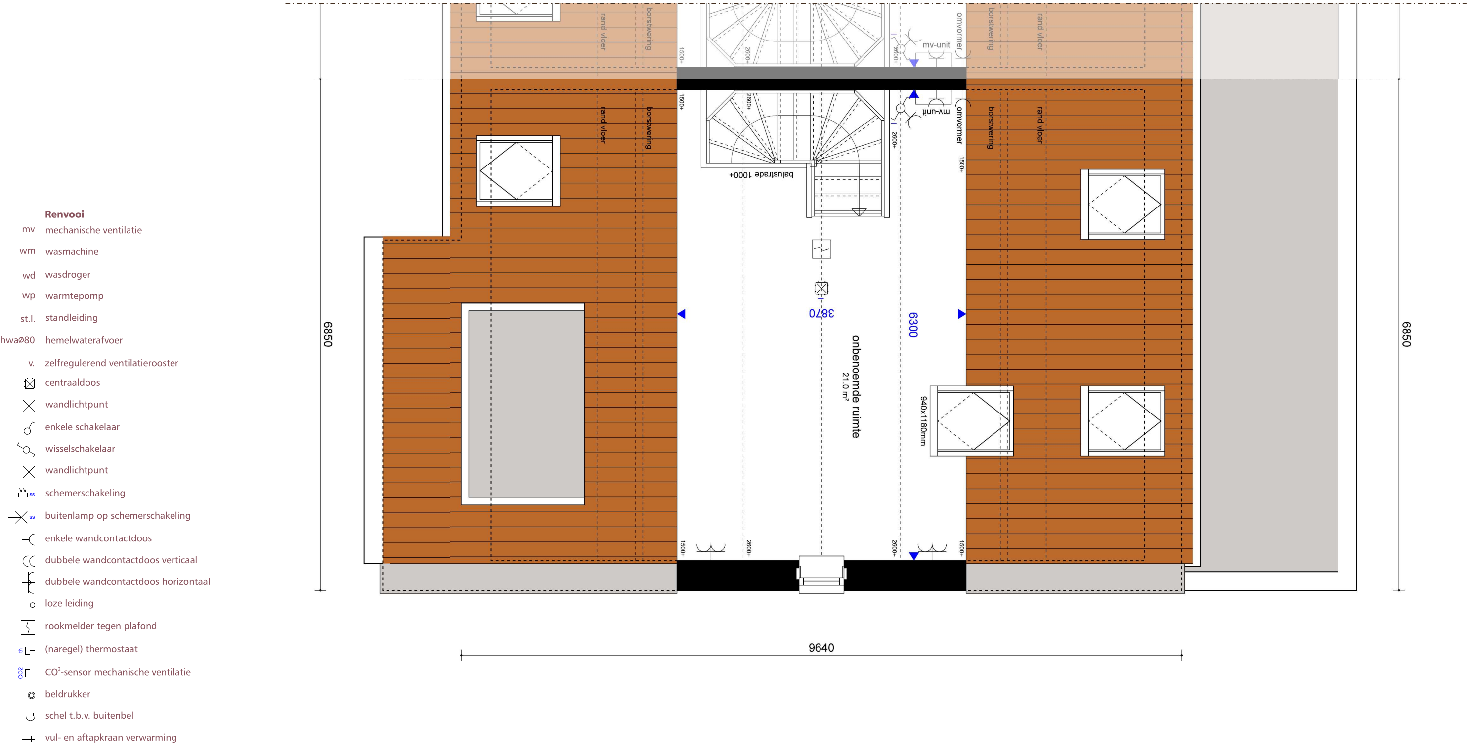
SCHAAL 1 OP 50 Plattegrond ~ Tweede verdieping
